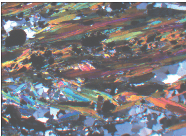
SEZIONE SOTTILE Micascisto granatifero, Punta Indren lato est
